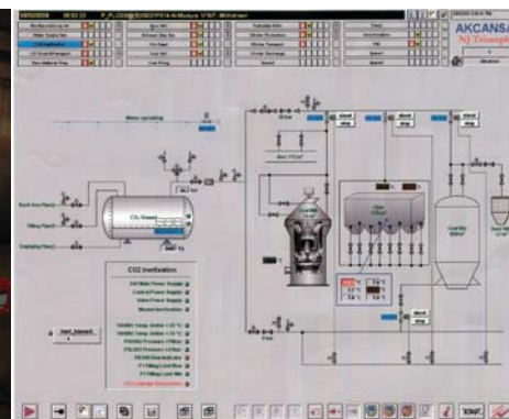
Рис. 1. Система CO 2 с резервуаром высокого давления и визуальным отображением на блоке контроллера PLC (цементный завод Akcansa - Canakkale компании Heidelberg Cement в Турции)
