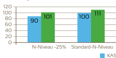
TM-Ertrag von Grünland relativ in Prozent
