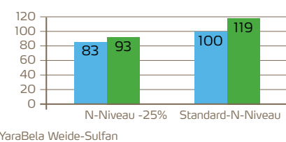
Protein-Ertrag von Grünland relativ in Prozent
